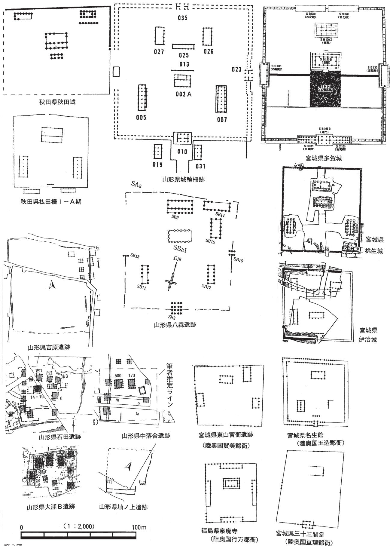
第3図 東北地方の主な正方形区画施設の建物模式図 (全て S = 1/2,000)
