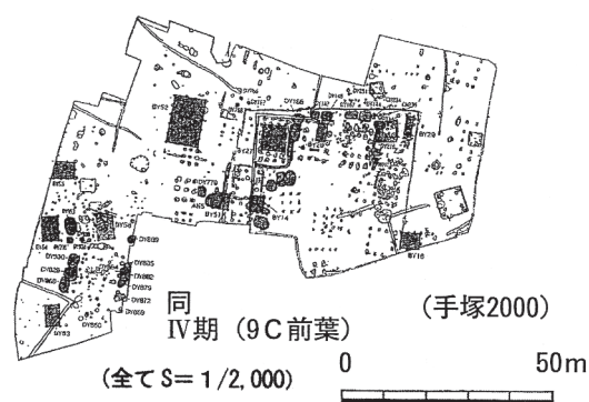
第4図 小規模区画施設遺跡の建物変遷図（1）
