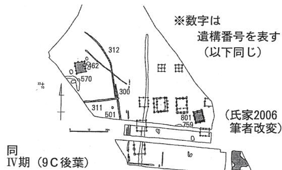
第5図 小規模区画施設遺跡の建物変遷図 (2) (全てS = 1/2,000)
