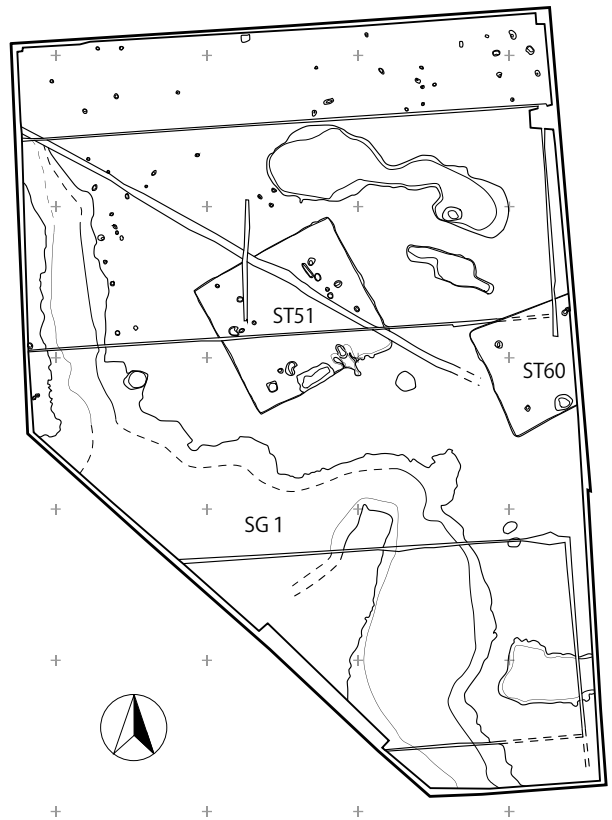
図1 遺構配置図 (S=1/400)
