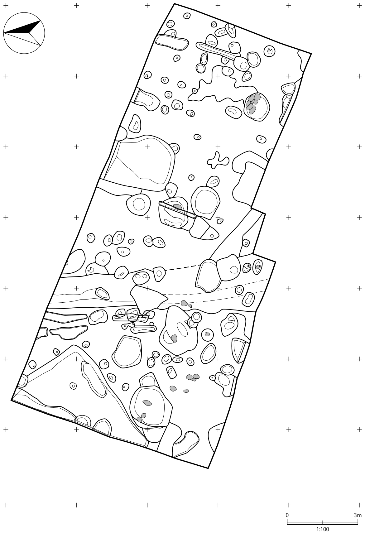
图2 P-4区遺構配置図 (S=1:100)
